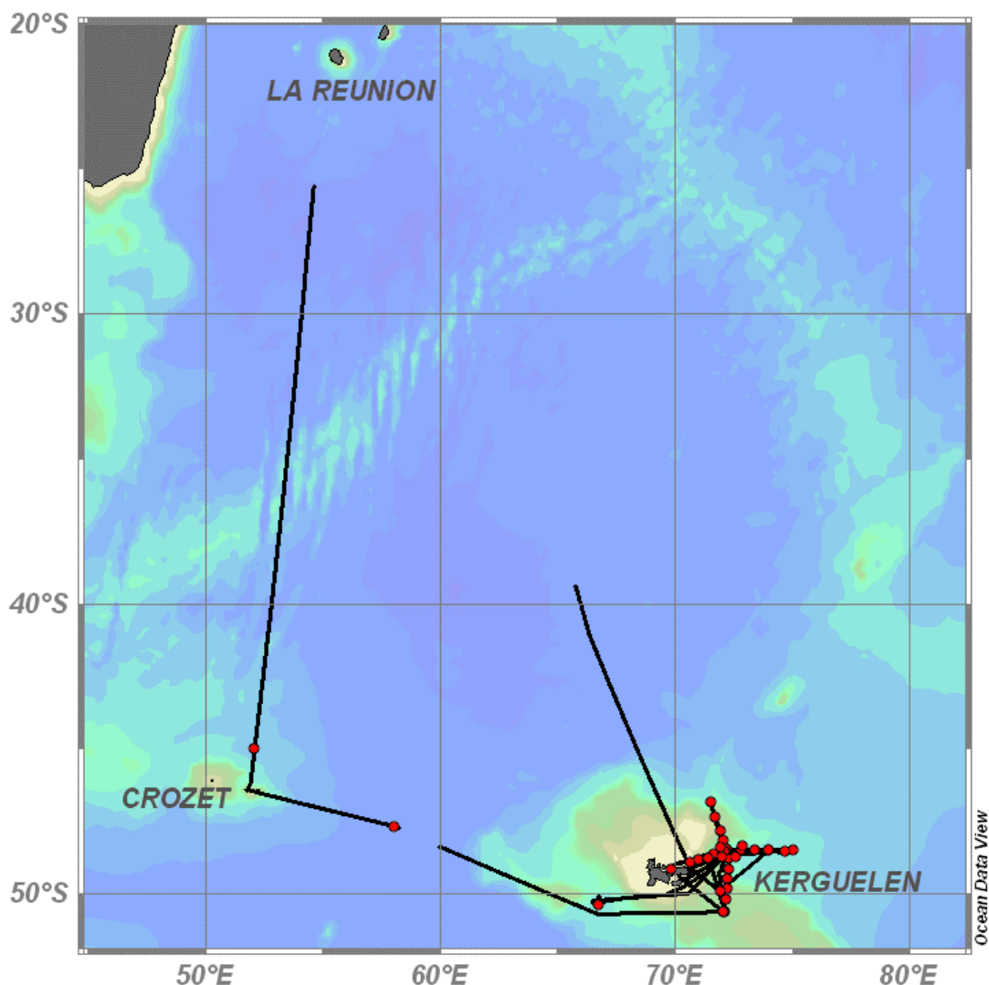
Carte situant les observations OISO acquises pendant la mission MD188/KEOPS2, dans les eaux de surface (mesures en continu, en noir) et dans la colonne d'eau (stations CTD, en rouge).
